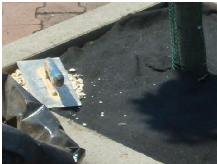
gyantával összekevert kavics kiöntése a geotextíliára, és a kiöntött anyag tömörítése
